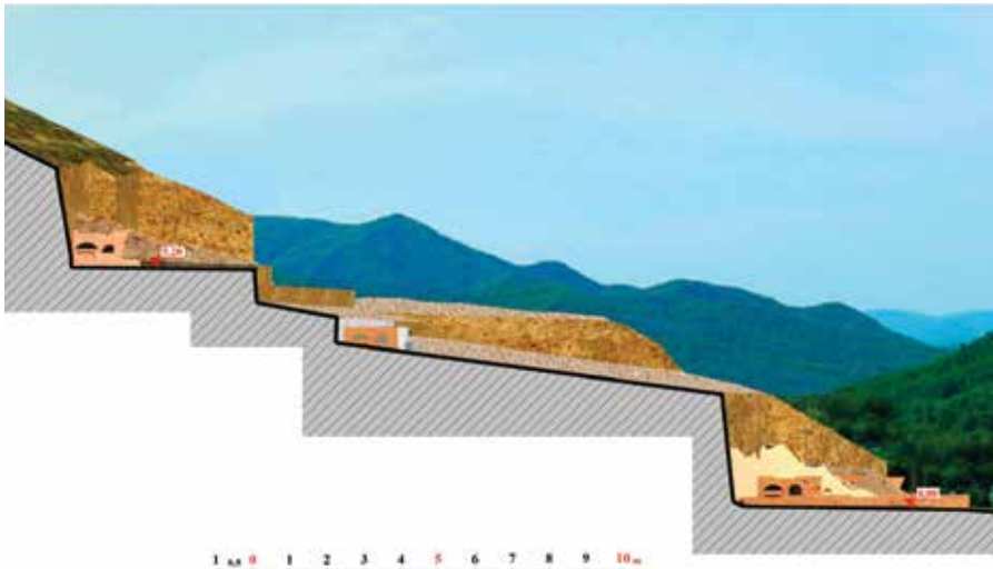
გრაკლიანი გორის III და IV ტერასის ნიშნულების პროფილი
